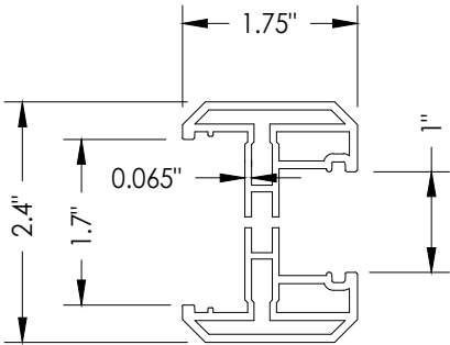
3A ODL LITE FRAME ALUMINUM
